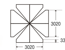
天幕(平面図)
